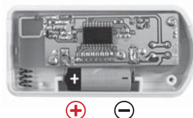
Rys.6 Polaryzacja baterii
