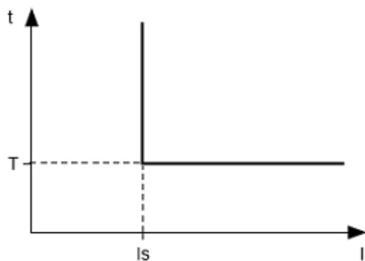
Rysunek 3.1 - Zasada działania zabezpieczenia zwłocznego niezależnego
